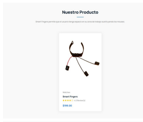
Figura 19. Página web
