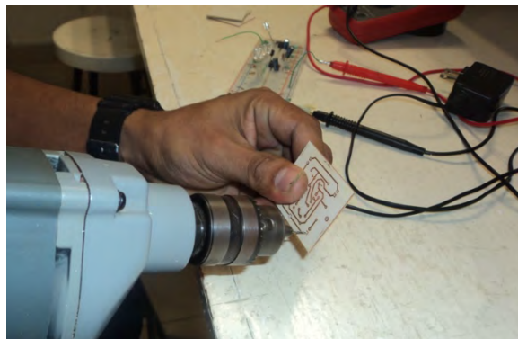
Imagen 15. Barrenado de circuito impreso del sensor electrostático.
