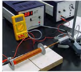
Figura 1.- medición de campo magnético creado por solenoide (en LT).
