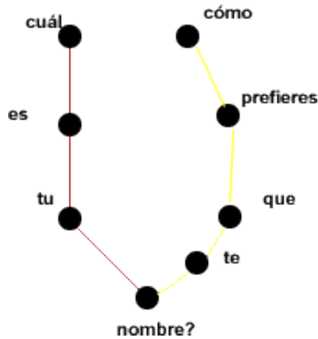
Figura 3. Grafo de decisión para diálogo en AIML (pattern).
