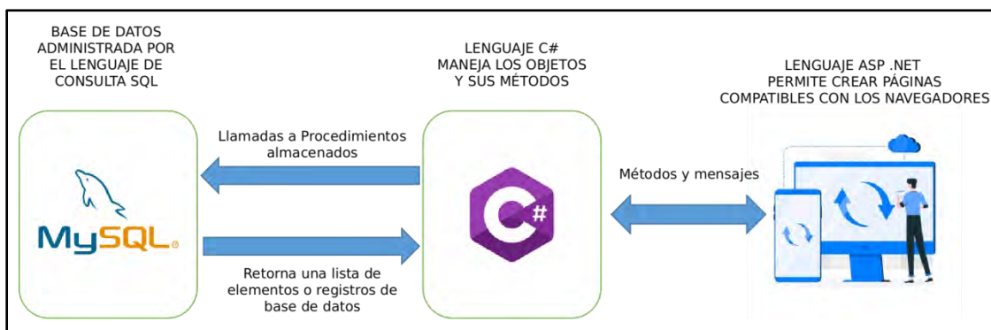
Figura 3. Estructura de la programación del sistema HJUDAS.
