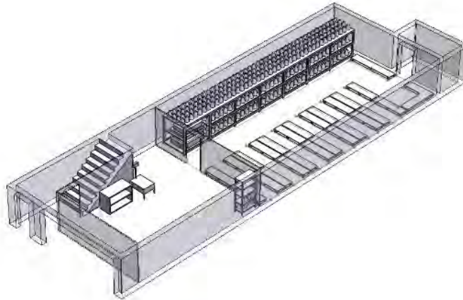
Figura 7. Visualización del almacén con pallets.
