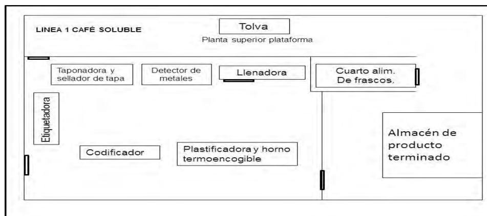
Figura 3. Distribución de línea / Fuente: propia del proyecto
