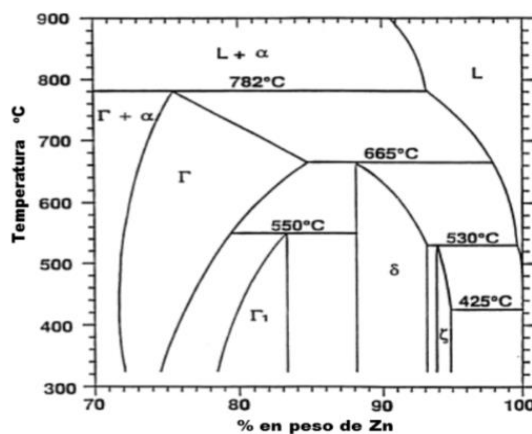
Figura 5. Diagrama de fases de equilibrio Zn-Fe ( Vera et al., 2013).
