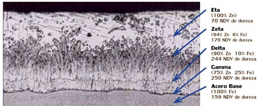
Figura 6. Microestructura del recubrimiento de zinc (Association americana galvanizers, 2015).
