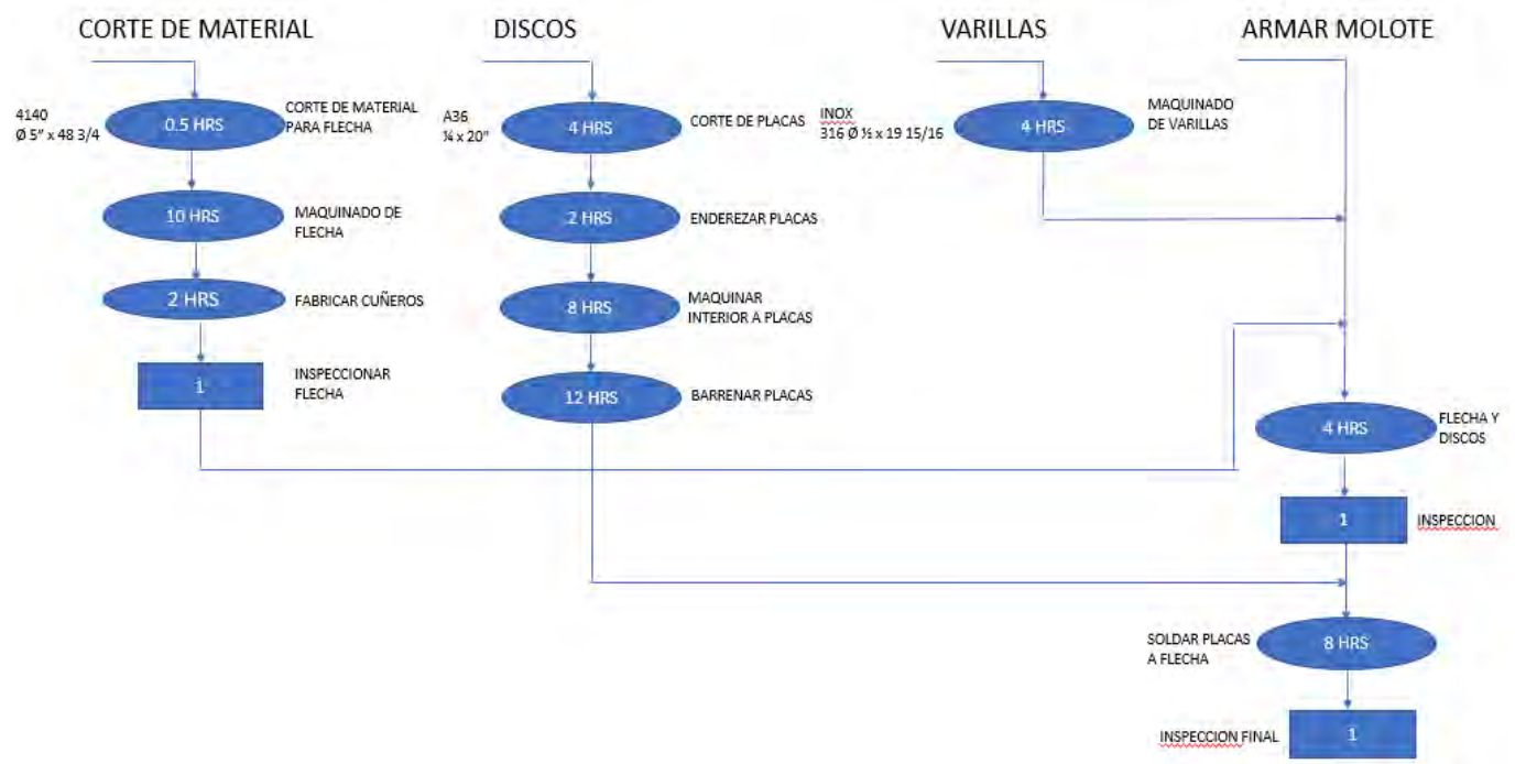
Figura 3. Modelo conceptual del proceso de fabricación del molote.
