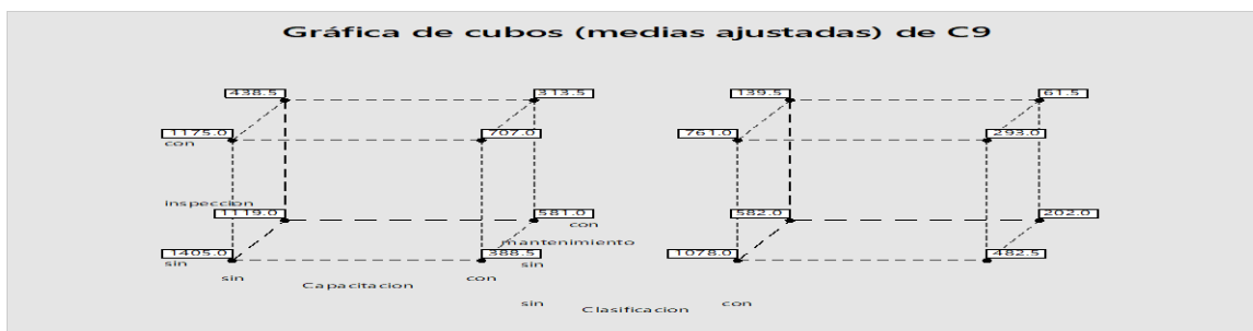
Figura 10: Gráfica de cubos
