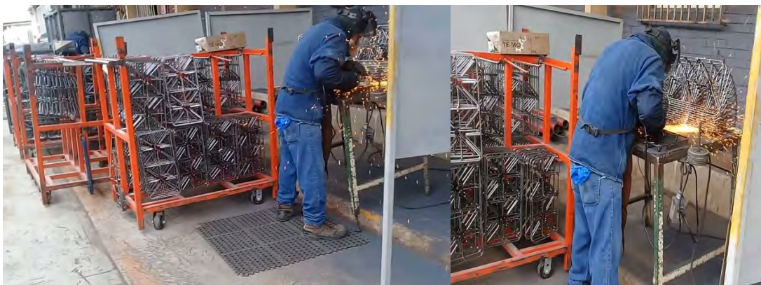
Fig. 10: Área de esmerilado
