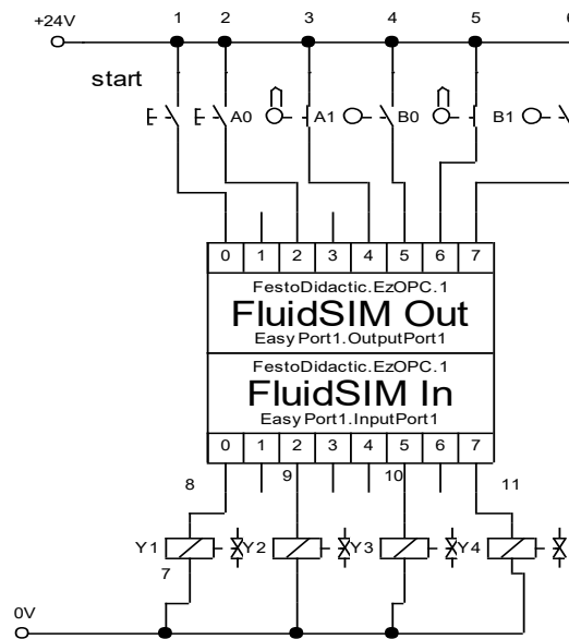
Figura No. 4 SIMULACION EN FLUIDSIM/CODESYS
