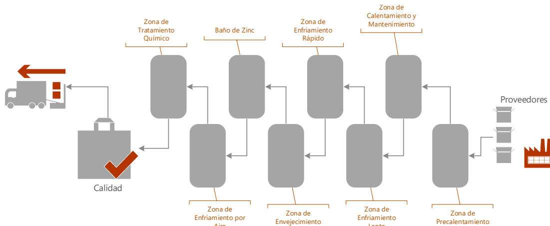
Figura. 1. Esquema básico de una línea de galvanizado en Caliente (LGC) (Adaptado de Martínez et al, 2007)
