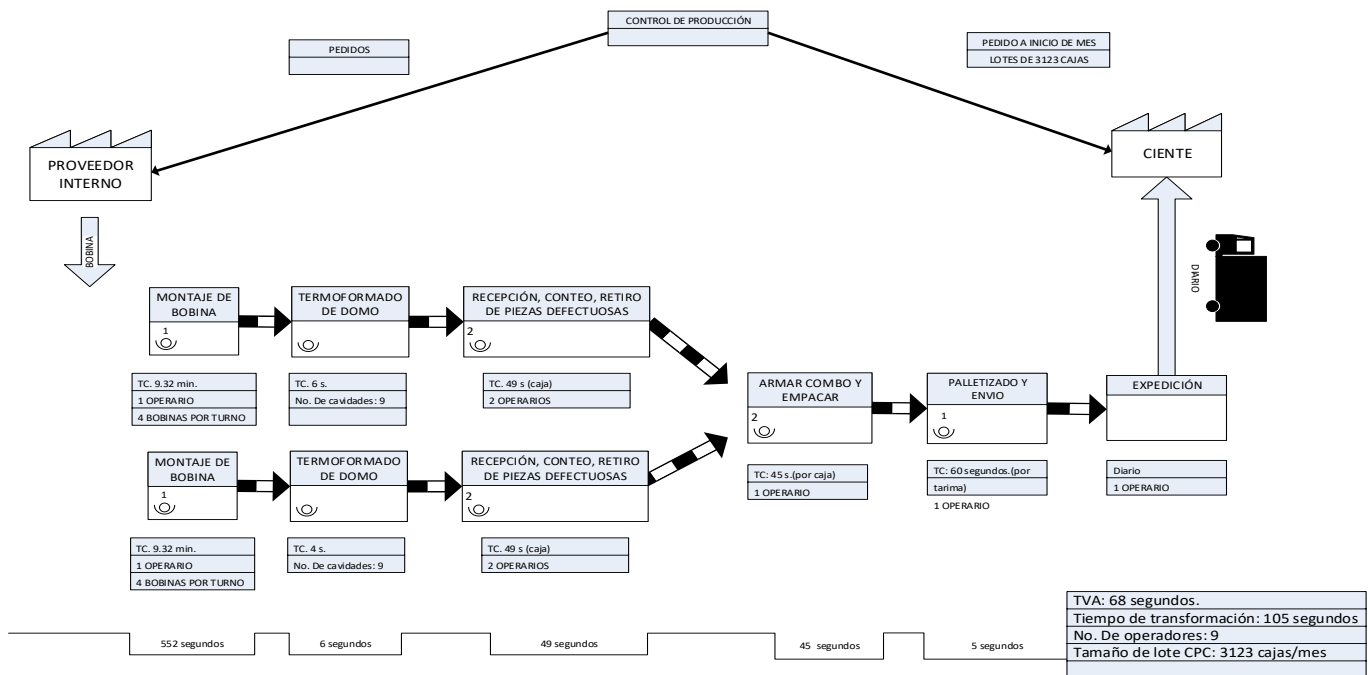
Mapa de cadena de valor VSM futuro.
