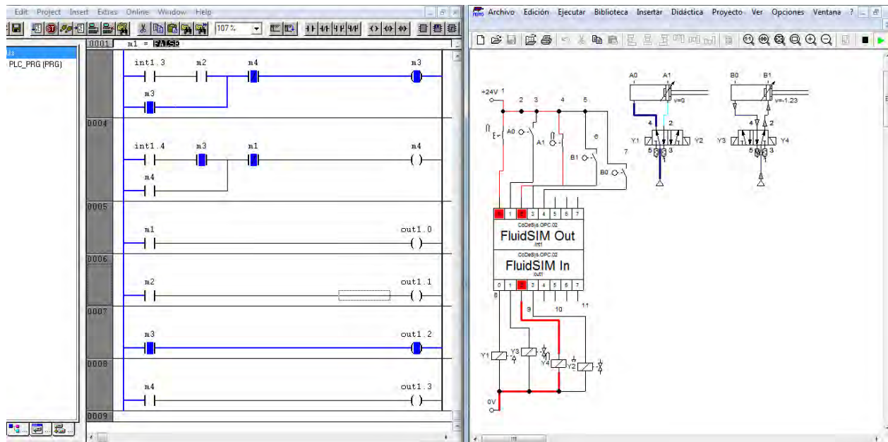
Figura No. 6 SIMULACION EN FLUIDSIM/CODESYS
