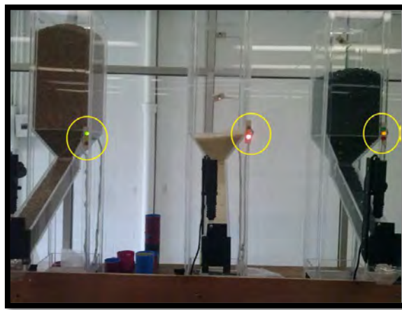
Imagen 4. Silos de granos en laboratorio CIM
