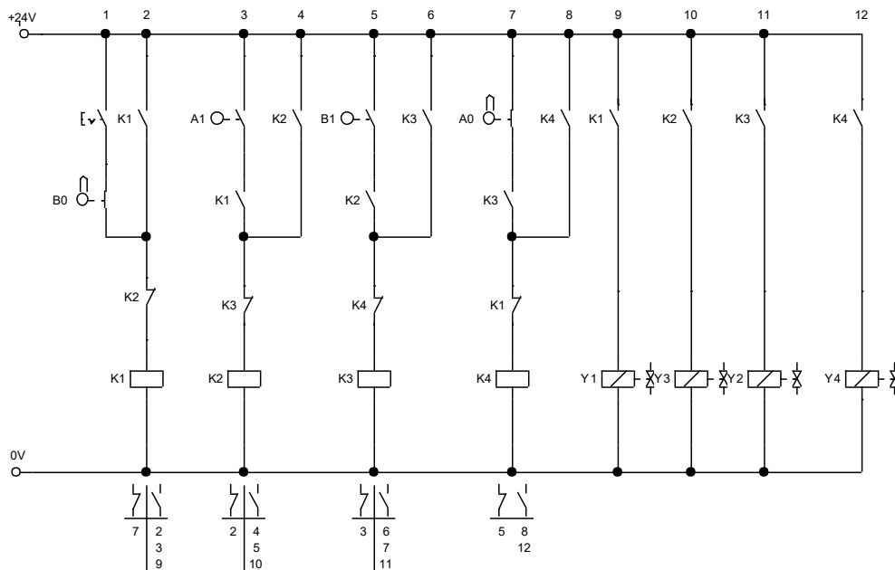
Figura No. 3 Diagrama electro neumático.
