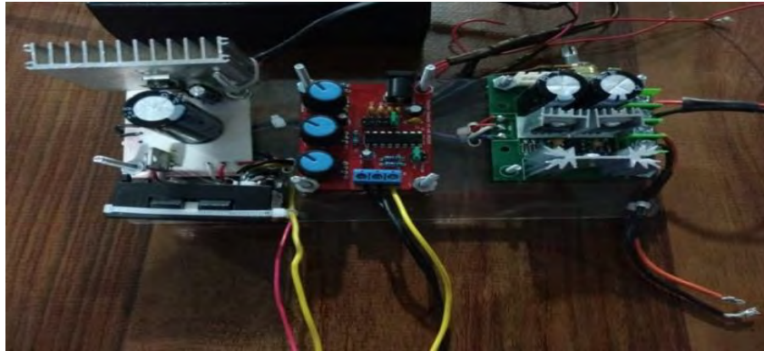
Figura 6. PWM, fuente y generador de ondas.
