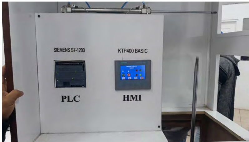
Figura No. 9 PRUEBA FINAL EN MODULO
