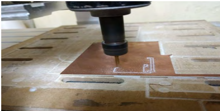
Figura 5. Manufactura con CNC.
