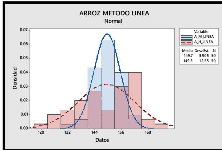
Imagen 14. Histograma Arroz método Línea
