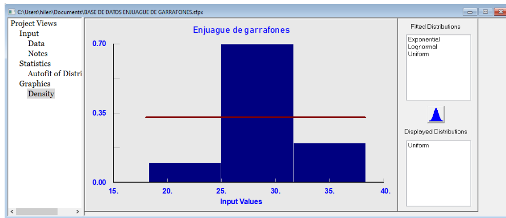
Figura 19.Histograma de la distribución de probabilidad uniforme para el enjuague de garrafrones.
