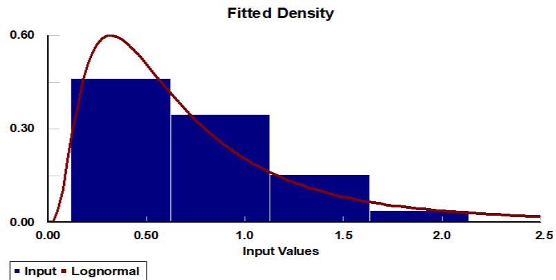
Figura 5. Tratamiento estadístico de la variable tiempo servicio en mostrador “comida”
