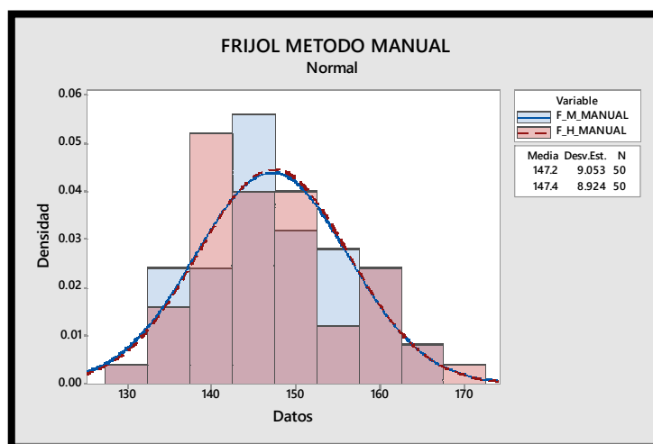
Imagen 9. Histograma Frijol método Manual
