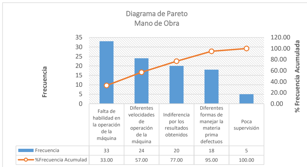
Figura 7. Diagrama de Pareto de la mano de obra.
