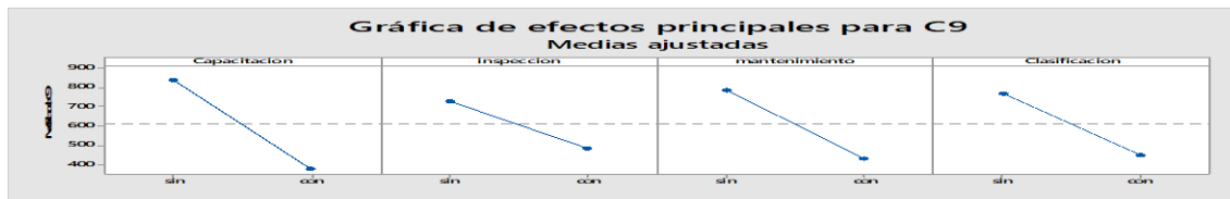
Figura 8: Gráfica de efectos principales
