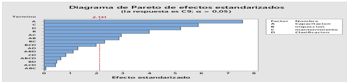
Figura 7: Diagrama de Pareto de efectos estandarizados
