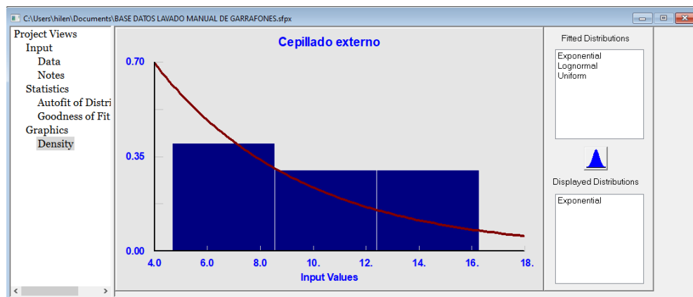
Figura 18. Histograma de la distribución de probabilidad exponencial para el cepillado interno de garrafones.
