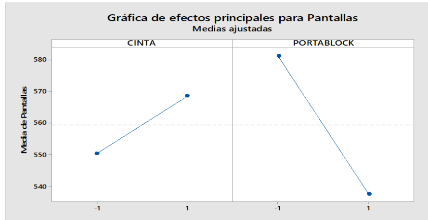
Figura 5. Gráficos de efectos principales
