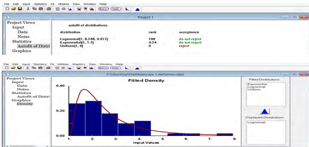
Ilustración 6. Análisis de la variable tiempo de atención en caja 3
