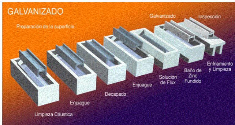
Figura 14. Etapas fundamentales en el proceso de galvanizado en caliente (Recuperado de S/N, 2019)
