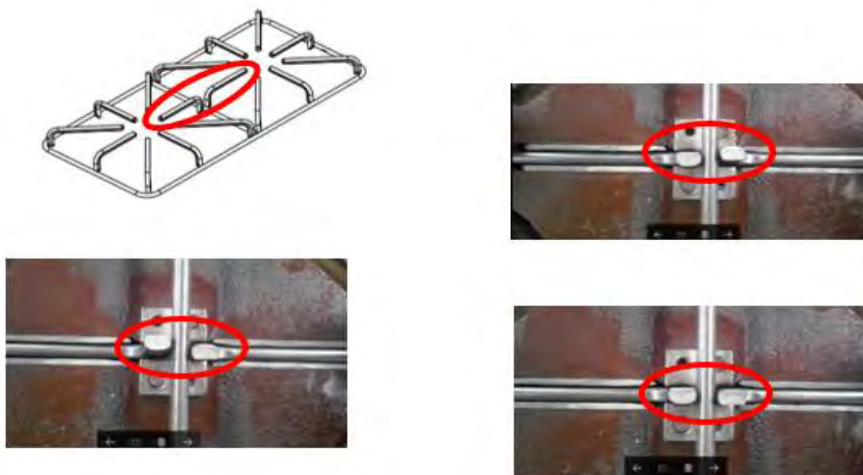
Fig.8: Situación actual de dedos centrales
