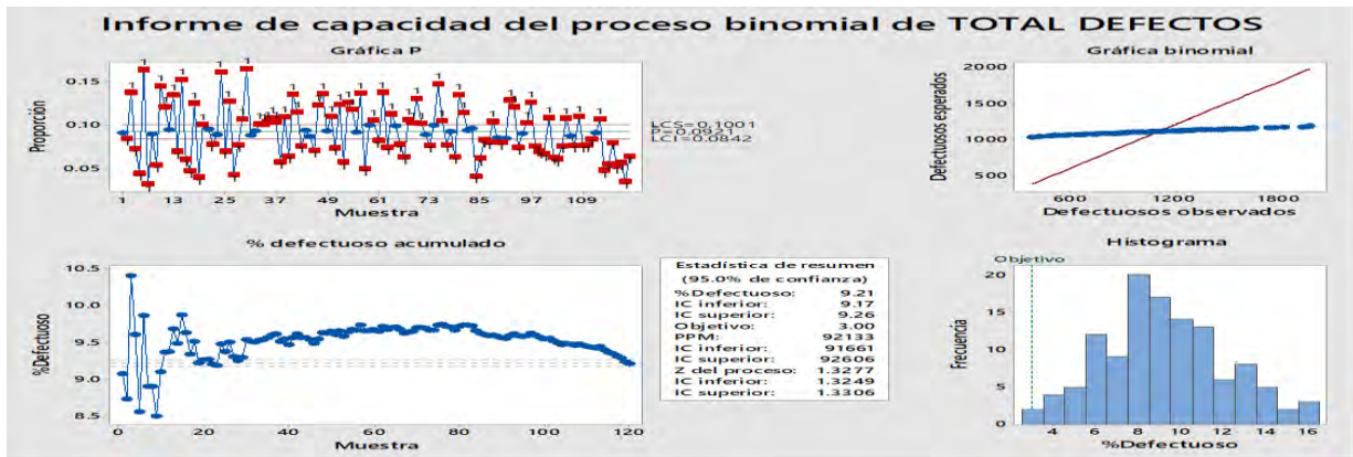
Figura 4: Informe de capacidad del proceso binomial de total defectos
