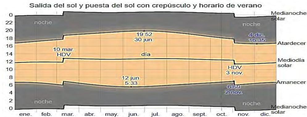
Figura 8. Comportamiento salida y puesta de sol con crepúsculo y horario de verano durante el año en el estado de Puebla
