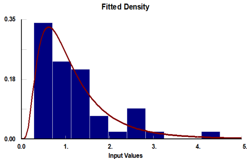
Figura 3. Tratamiento estadístico de la variable tiempo servicio en mostrador “producto mostrador”
