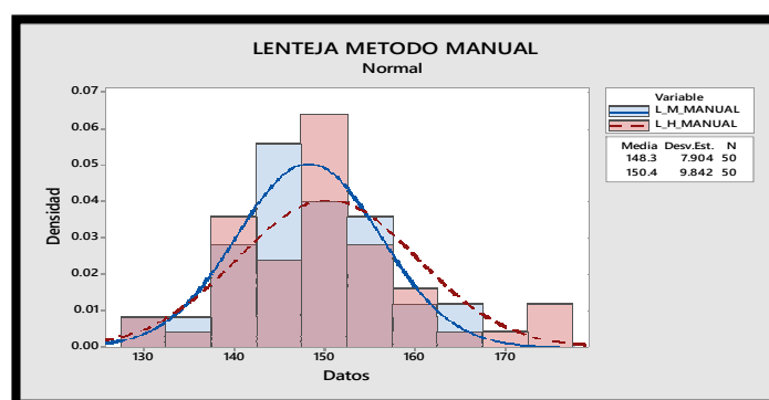
Imagen 8. Histograma Lenteja método Manual
