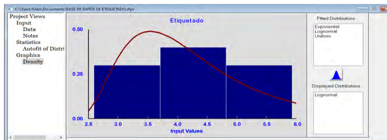
Figura 22.Histograma de la distribución de probabilidad lognormal para el etiquetado de garrafones.
