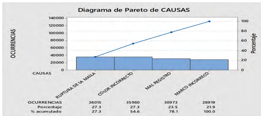
Figura 2: Diagrama de Pareto
