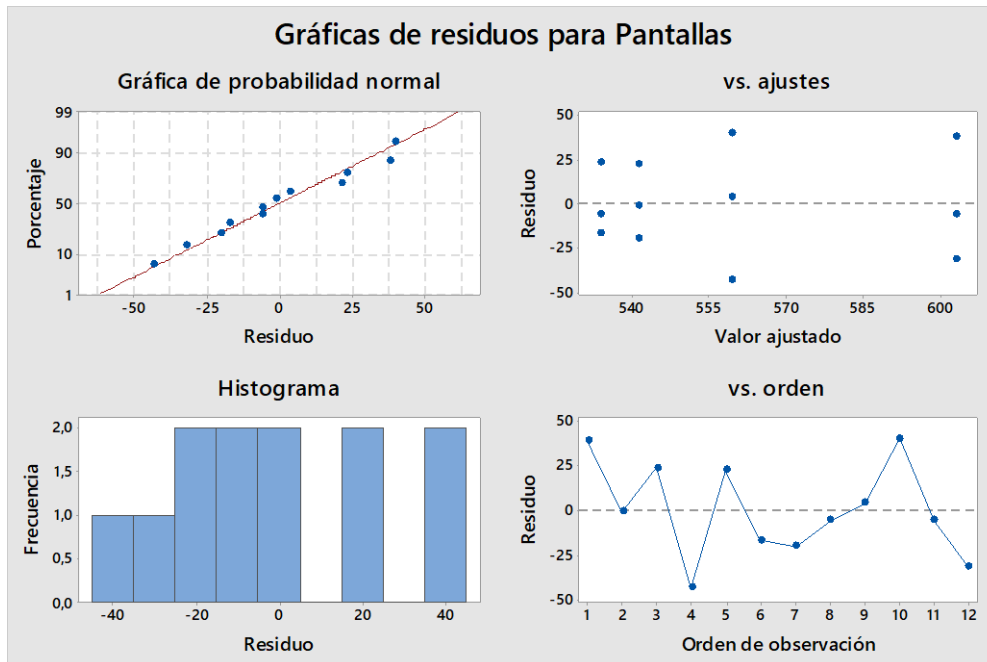
Figura 3. Gráficos de residuos para pantallas rotas
