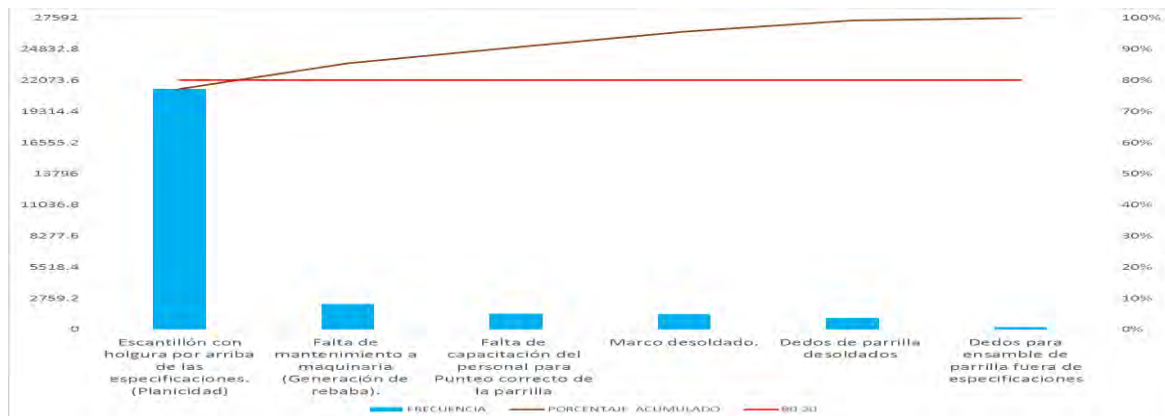
Fig. 4: Diagrama de Pareto
