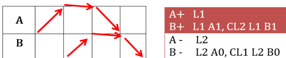
Figura No. 2 Diagrama de espacio-fase
