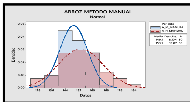
Imagen 7. Histograma Arroz método Manual
