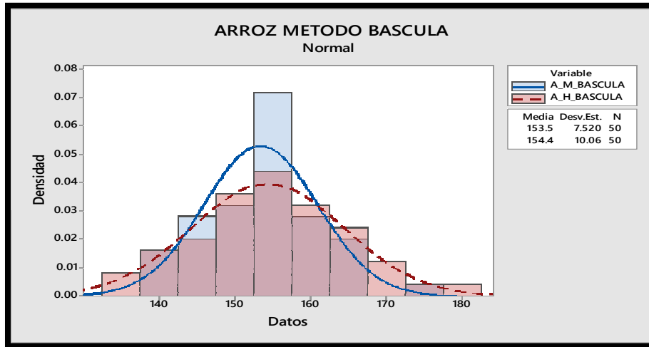
Imagen 21. Histograma Arroz método bascula
