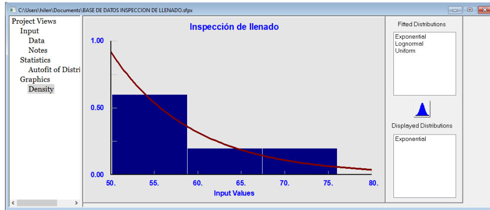
Figura 21.Histograma de la distribución de probabilidad exponencial para la inspección de llenado en garrafones.
