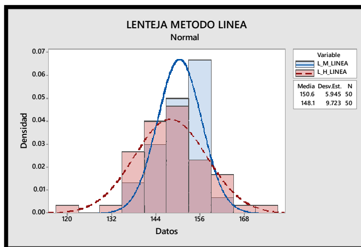
Imagen 15. Histograma Lenteja método Línea
