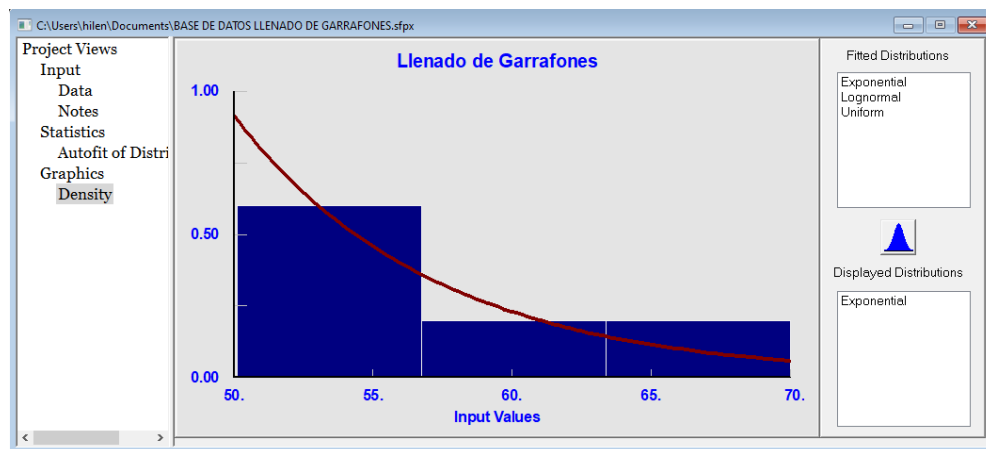
Figura 20.Histograma de la distribución de probabilidad exponencial para el llenado de garrafrones.
