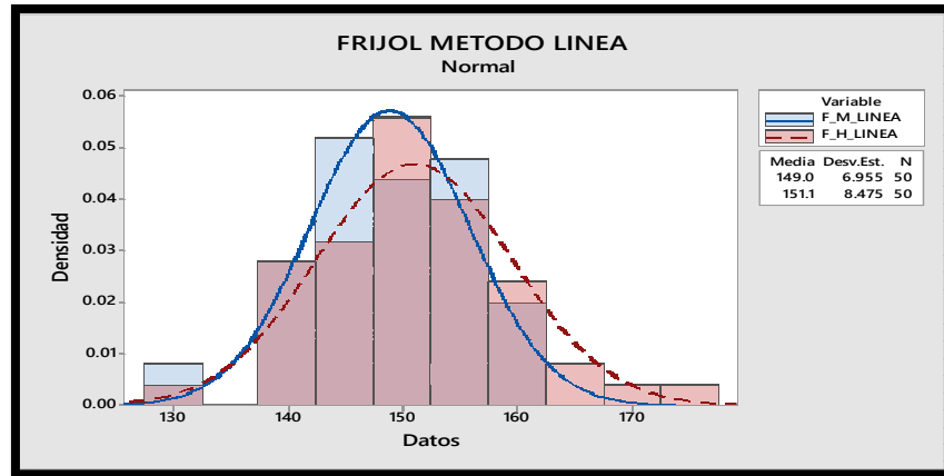
Imagen 16. Histograma Frijol método Línea
