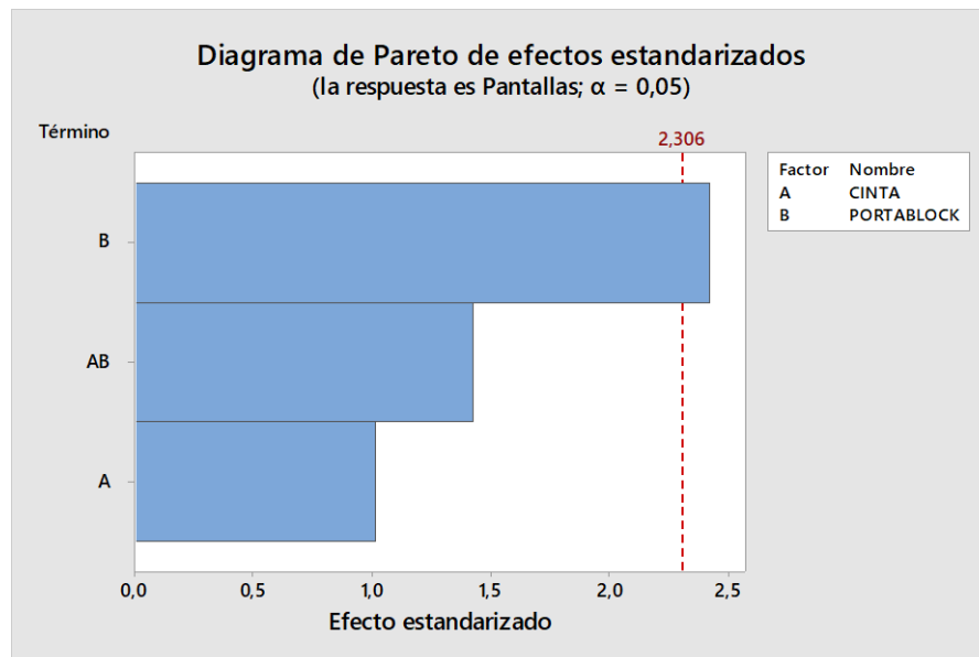
Figura 4. Diagrama de Pareto de efectos estandarizados
