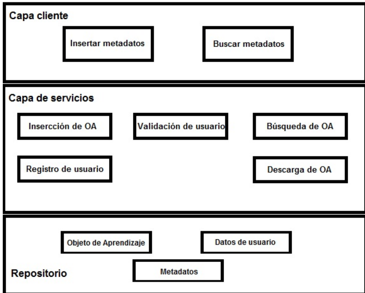
Figura. 4.- Arquitectura del sistema.
