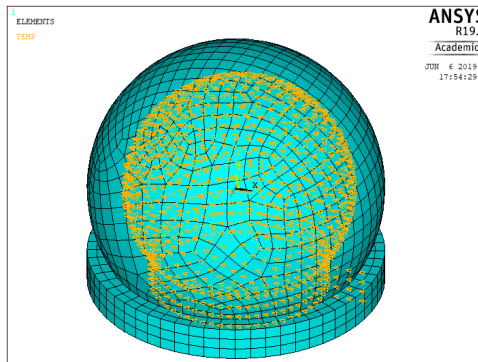
Figura 6. Aplicación de cargas por temperatura en el horno.
