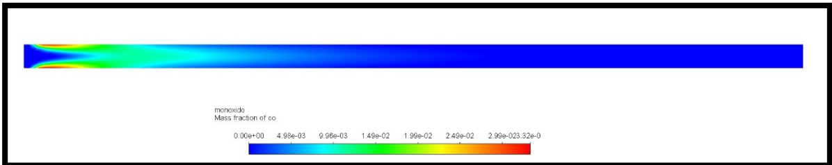
Figura 13. Contorno de la fracción másica del monóxido de carbono como producto de las reacciones en el sistema.
