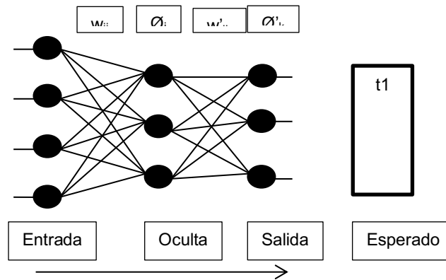
Figura 3. Arquitectura unidireccional con tres capas
