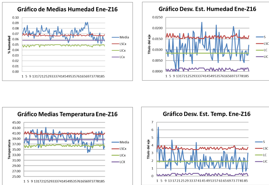
Gráficos X-S humedad y temperatura zafra 2016
