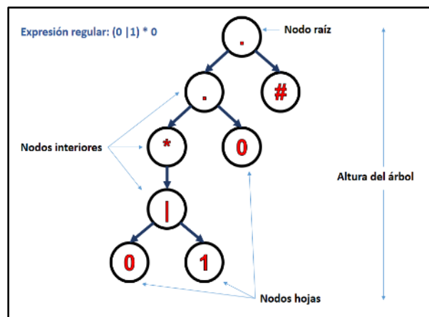
Figura 3. Elementos que conforman el árbol sintáctico
