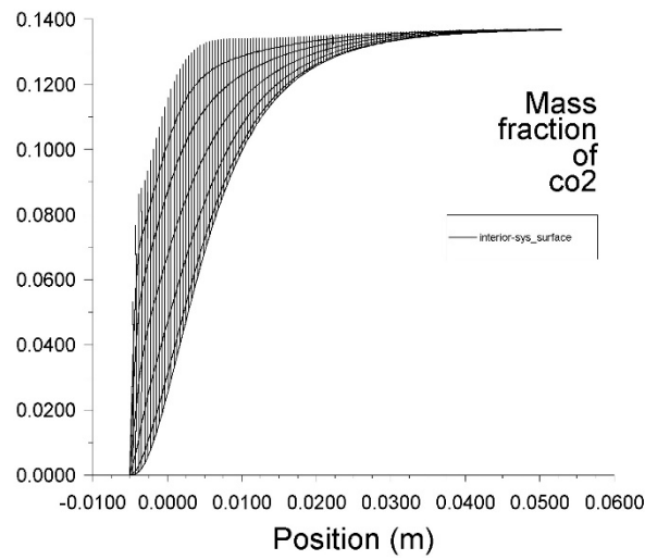
Figura 21. Gráfica de la posición en X contra la fracción másica de monóxido de carbono producido.
