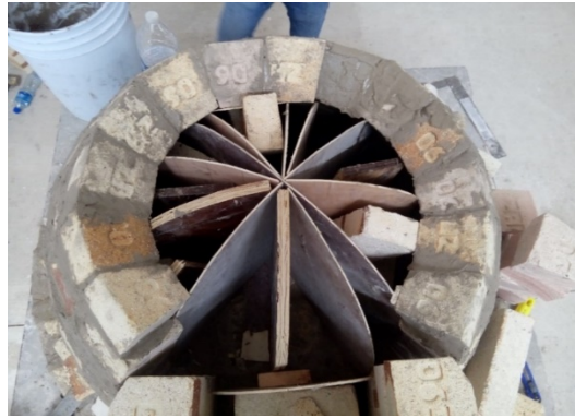
Figura 13. Cimbra para la construcción del domo del horno
