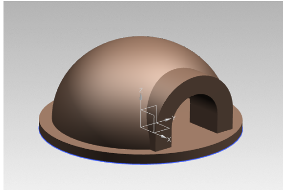
Figura 5. Diseño final de horno tipo domo.
