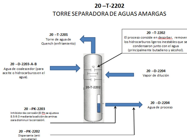
Figura No.1.Torre 20-T-2202 Torre separadora de aguas amargas
