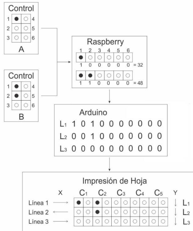
Figura 9. Proceso del sistema de impresión braille.
