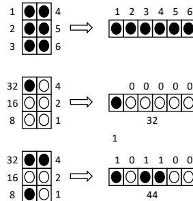
Figura 7. Conversión de Braille a bytes
