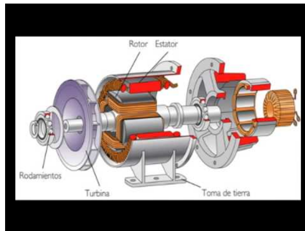
Figura 3.- Partes que constituyen el Generador electromagnético
