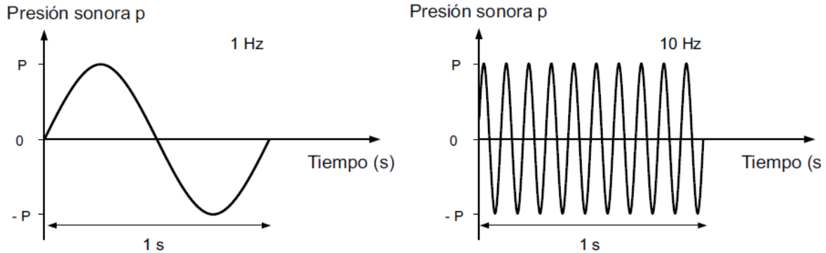
Figura 2. Comparación de una onda de 1 Hz y 10 Hz (Carrión, 1998)
