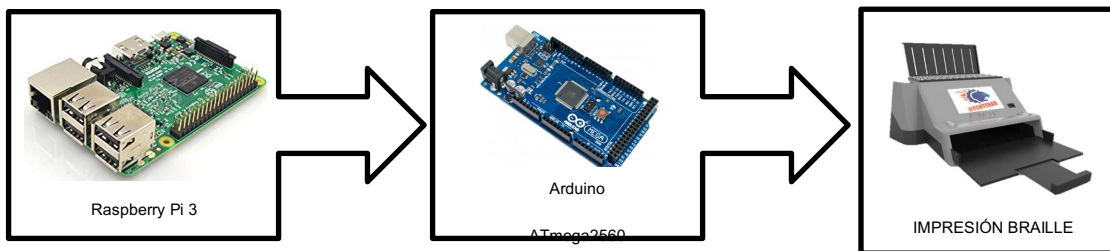
Figura 5. Esquema general de control de impresión Braille
